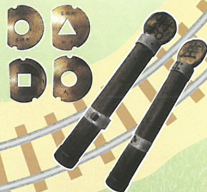
松電の通票(タブレットとスタッフ) (松阪市文化財センター蔵)
